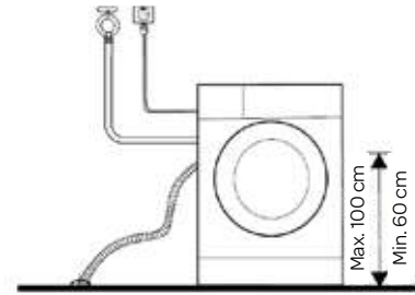
1. In einen Bodenablauf gesteckter Wasserablaufschlauch.
