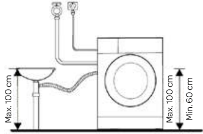
2. An ein Abflussrohr angeschlossener Wasserablaufschlauch.
